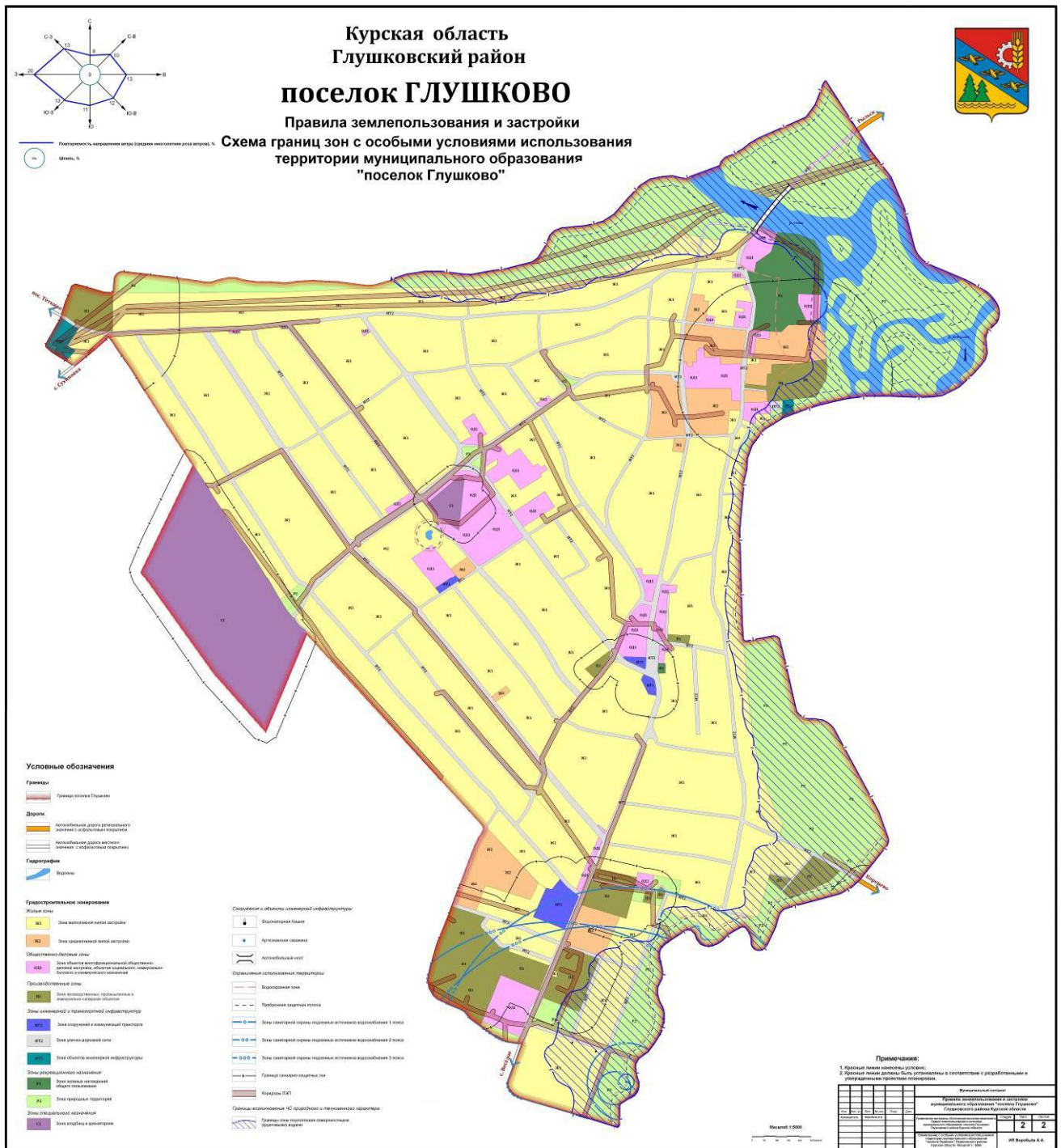
Рис.2. Схема границ зон с особыми условиями использования территории муниципального образования «поселок Глушково» Глушковского района Курской области
